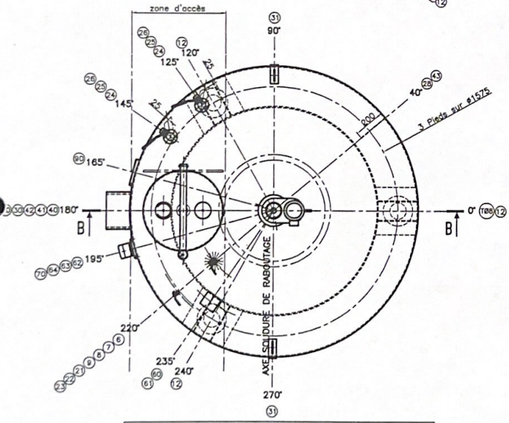
VUE EN ORIENTATION SEULE LA VUE DE DESSUS EST VALABLE POUR LES ORIENTATIONS
