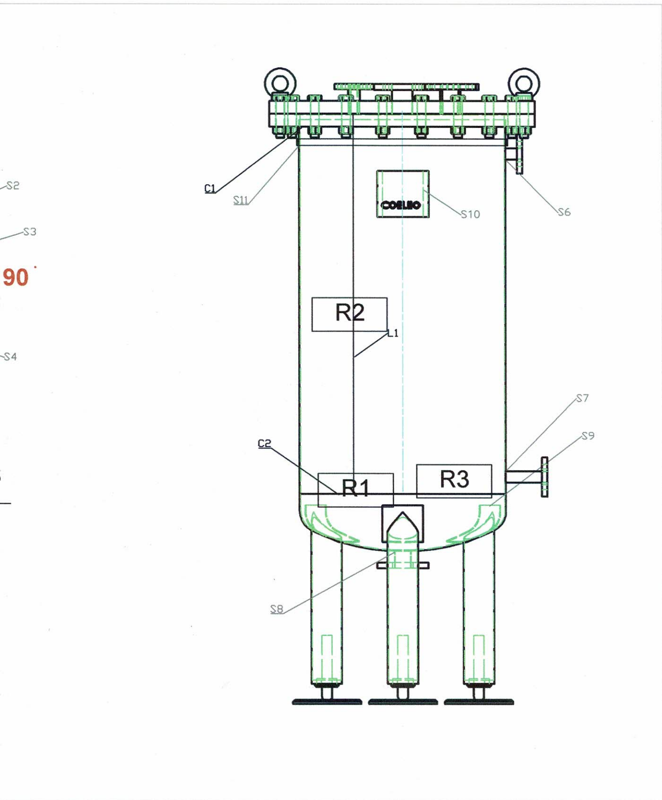
Appareil Protégé par une Soupape Tarée à 2B
