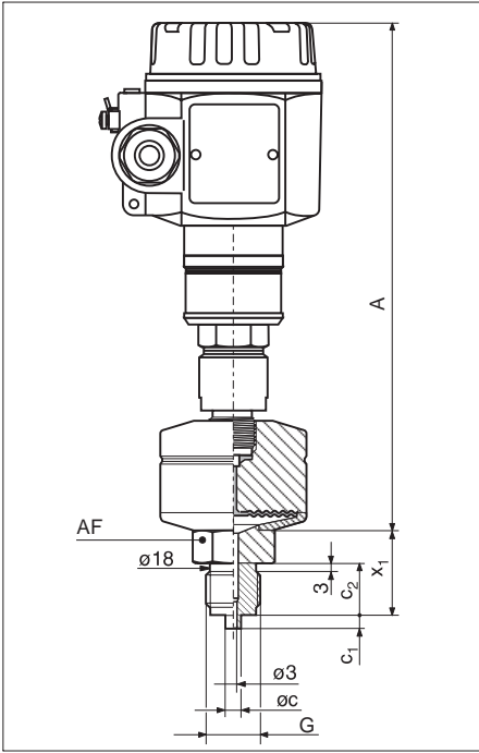
Separator with G ½ A; EN 837 Form B 6kt
