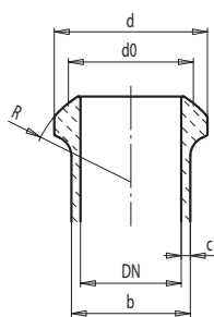
KF-Kugel Schott
