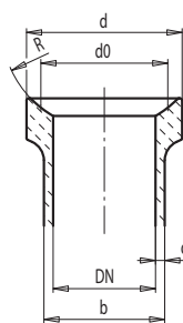
KF-Pfanne Schott
