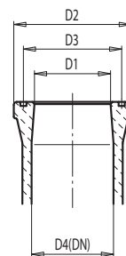
Planflansch QVF
