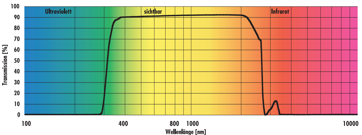
Transmissionskurve Borosilicatglas
