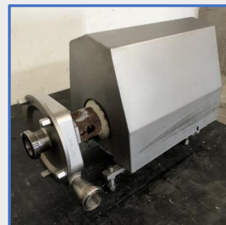
TUCHENHAGEN 7,5 KW Centrifuge inox S/s centrifuge pump
