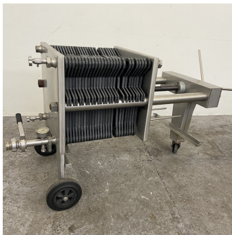
Filtre à plaques 385 x 385 mm Filter press
