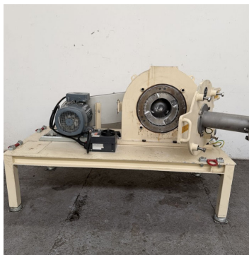
Broyeur à impact 11KW BAUERMEISTER type UMT1.3EX Impact mill
