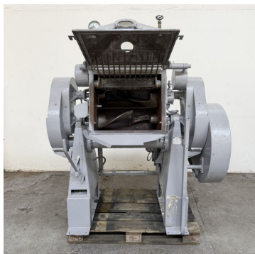
Malaxeur à 2 bras en Z 85L GUITTARD type M53L 2 arm Z-shaped kneader mixer
