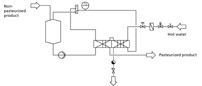
P&I Diagram
